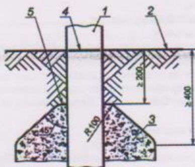
1 — опора; 2 — поверхность покрытия игровой площадки; 3 — фундамент; 4 — базовая отметка заглобления; 5 — верх фундамента
